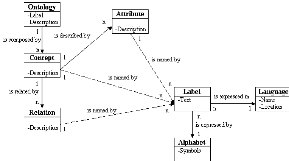
Figura 16: Ejemplo de metamodelo de multilingüidad para etiquetas de conceptos, de atributos y de relaciones
