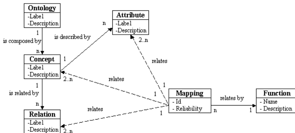
Figura 17: Ejemplo de metamodelo de multilingüidad con mappings para etiquetas de conceptos, de atributos y de relaciones
