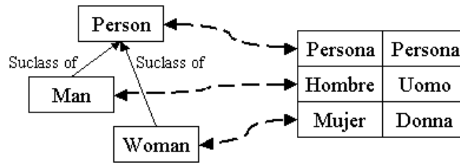
Figura 22: Ejemplo de modelo basado en un metamodelo de multilingüedad con metamodelo de ontologías monolingües y modelo de recurso lingüístico
